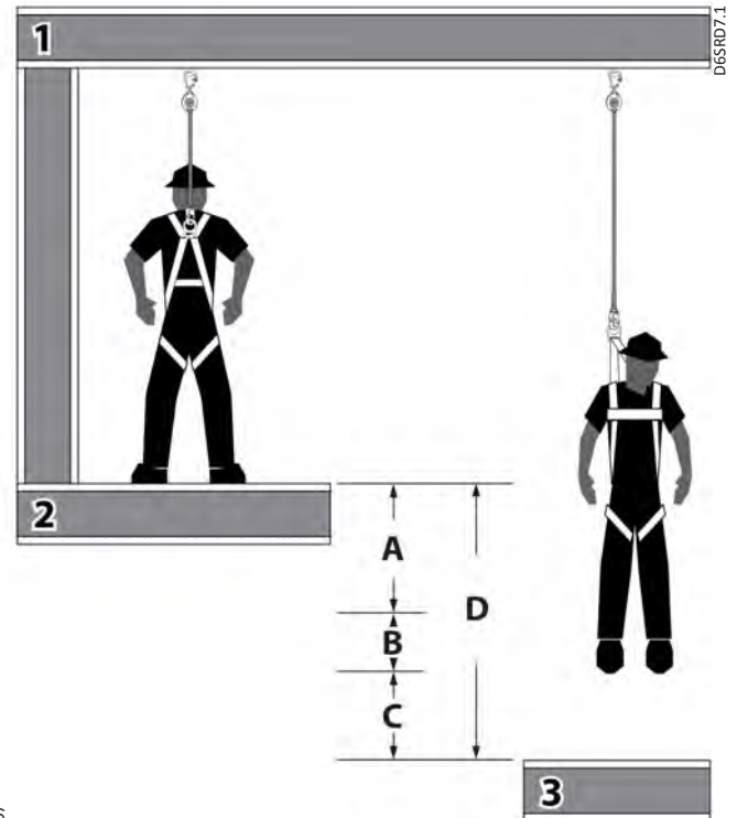
Fig. 3A: Distancia mínima de caída despejada requerida - SRD de 6 pies (1,8 m)
