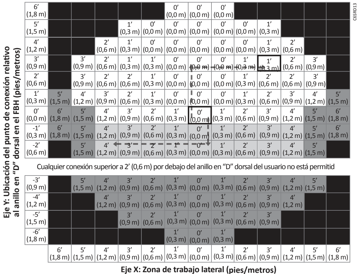
Gráfico 1: Distancia despejada de caída adicional requerida debido a la caída con balanceo (pies/metros)
