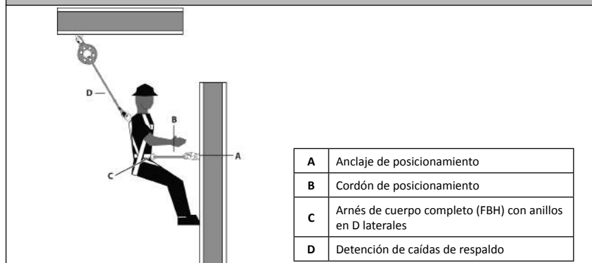
Figura 8 - Posicionamiento de trabajo
