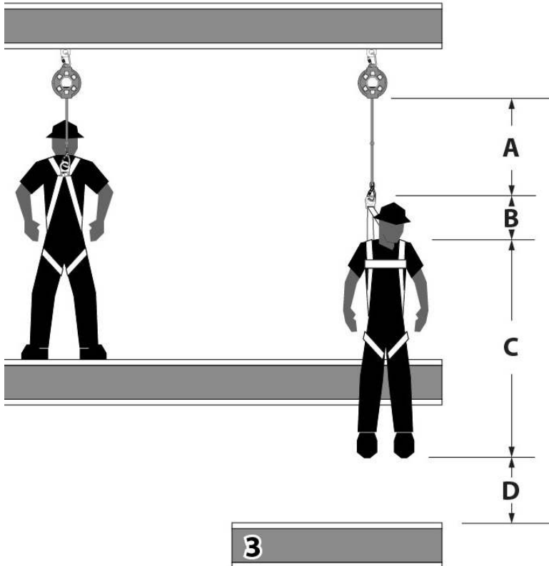
Figura 4 - Requisito mínimo de caída despejada: cuerda autorretractil ANSI Clase B
