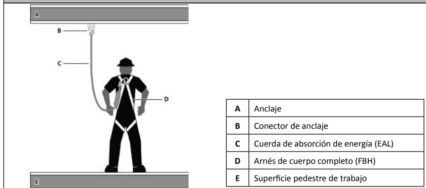
Figura 7 - Detención de caídas (PFAS)
