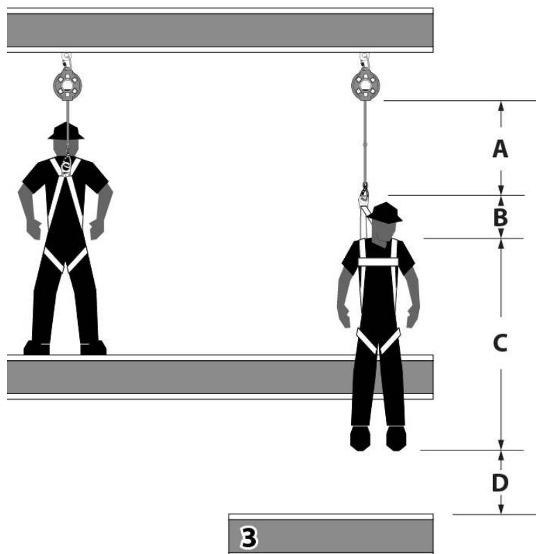
Figure 4 - Dégagement minimal requis en cas de chute : Cordon à rappel automatique, ANSI Classe B
