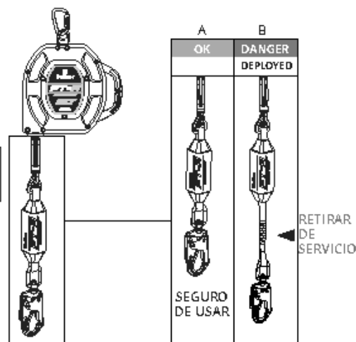
Figura 8 - Inspección del absorbedor de energía indicador de carga del SRD
