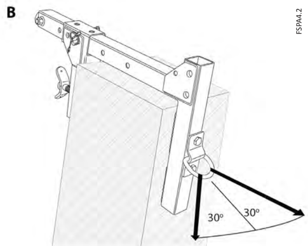
Fig. 4: Dirección de la carga y rango de trabajo
