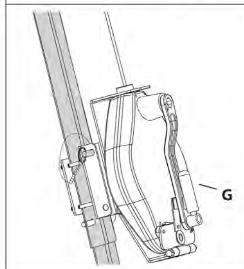
Figura 5B: Conecte la SRL de recuperación al soporte de la pata
