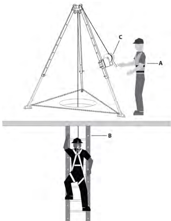
Figura 2A: Uso del trípode con cabrestante únicamente
