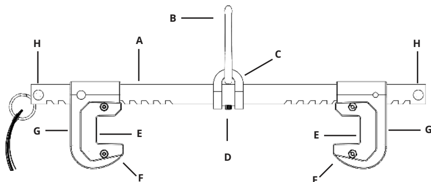
Figura 1 - Acerca del Anclaje Beam de FallTech®
