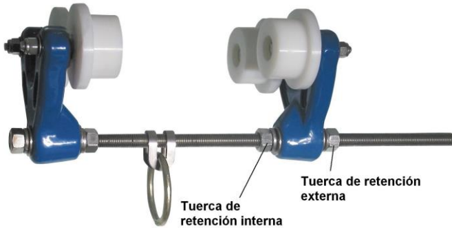
Fig. 3.7 Carrito de viga de FallTech (7710)
