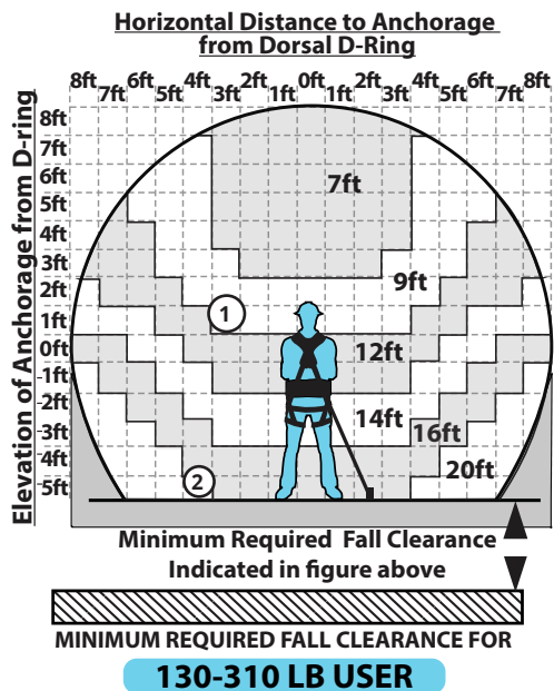
Figure 11 - Dégagement de chute minimum requis pour le CT-X pour les utilisateurs de 59 à 141 k (130 à 310 lb)
