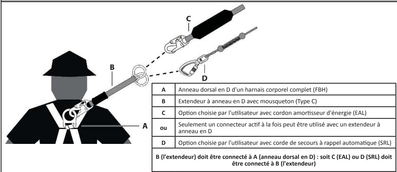
Figure 9 : Utilisation convenable de l'extendeur à anneau en D de Type C
