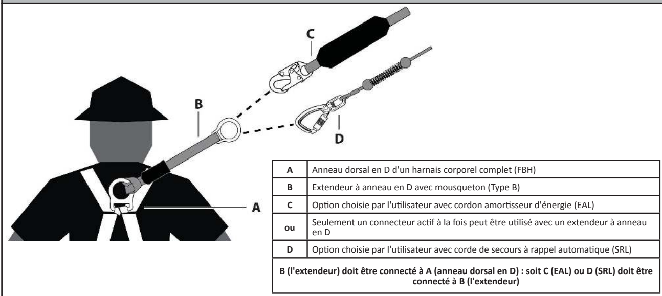
Figure 8 : Usage adéquat d'un extendeur à anneau en D de Type B
