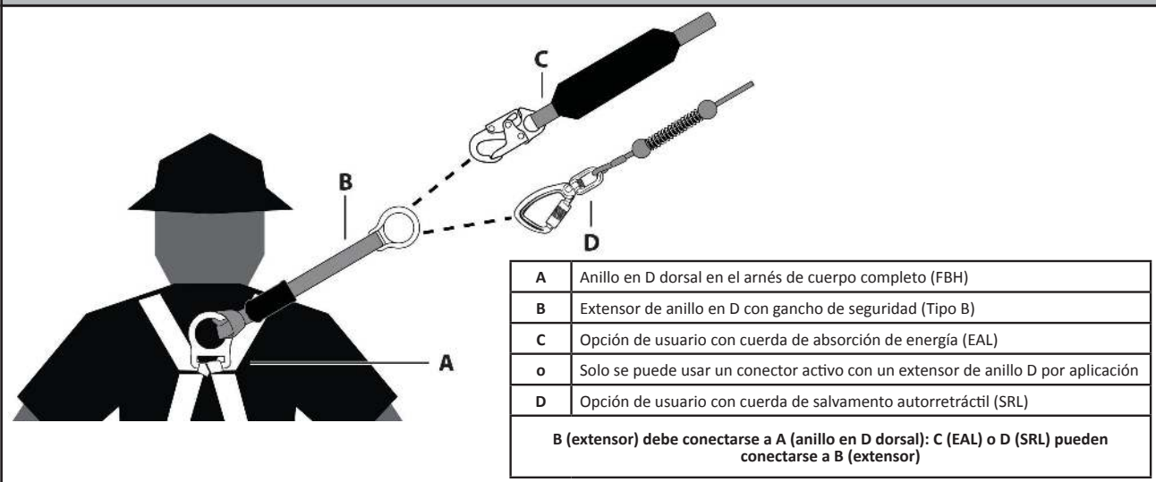
Figura 8: Uso adecuado del extensor de anillo en D tipo B
