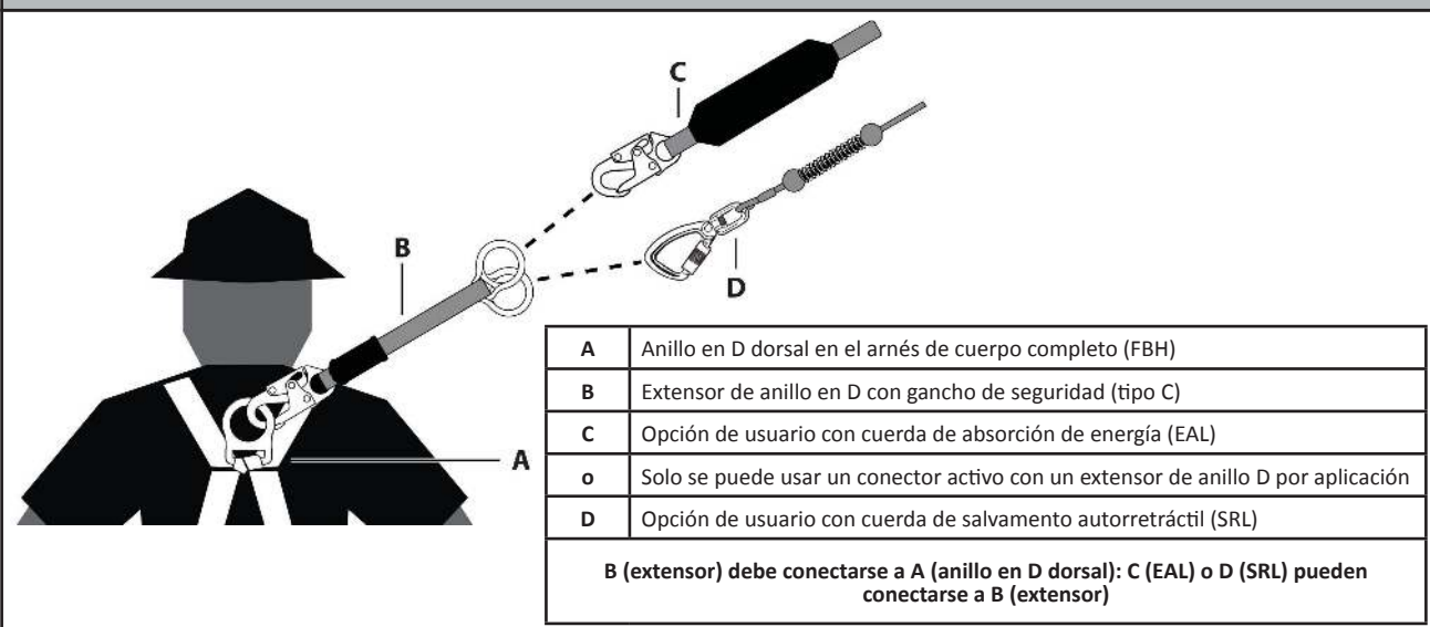
Figura 9: Uso adecuado del extensor de anillo en D tipo C
