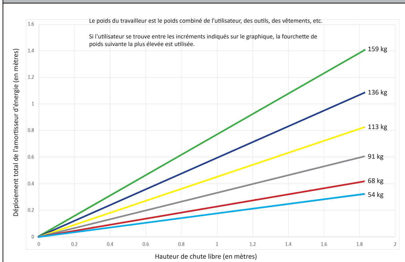
Graphique 1 - Déploiement du cordon amortisseur d'énergie
